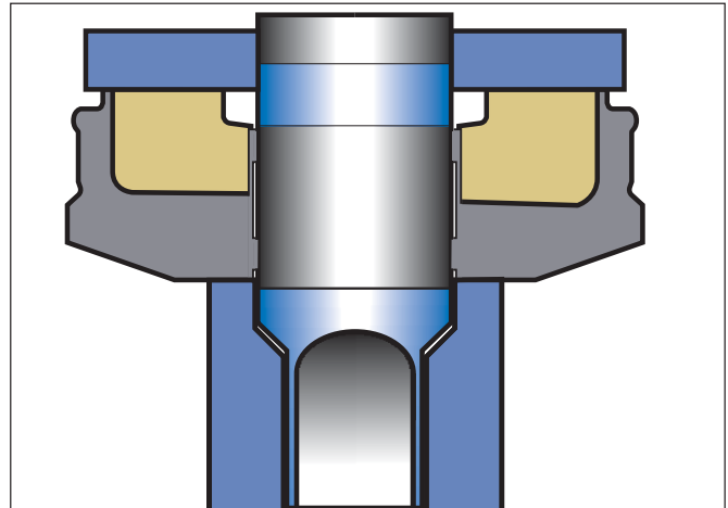
Dry stem journal.
