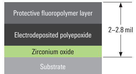
ZPEX layer composition.
